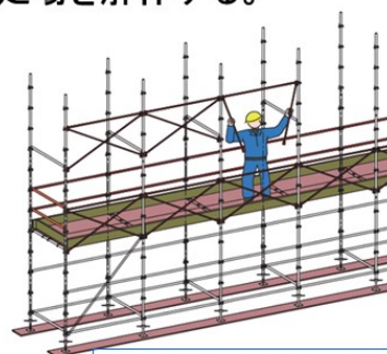
くさび緊結式足場の例
